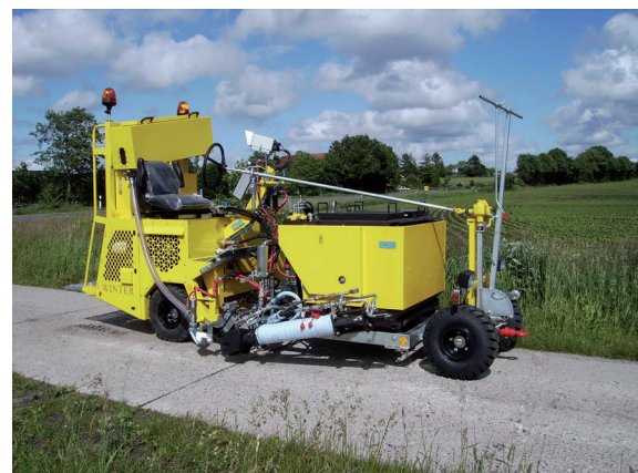
ekstruder do mas termoplastycznych
